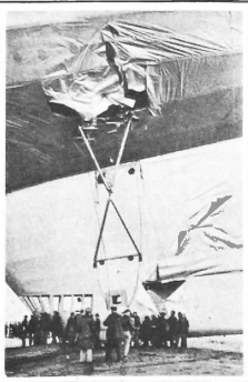
Al intentar su primer vuelo de prueba, el "Akron" fue lanzado contra el suelo, sufriendo serios daños. Este primer accidente demostró la debilidad original de su estructura. Véanse las averías producidas en el involucro por un ligero choque de la barquilla.
